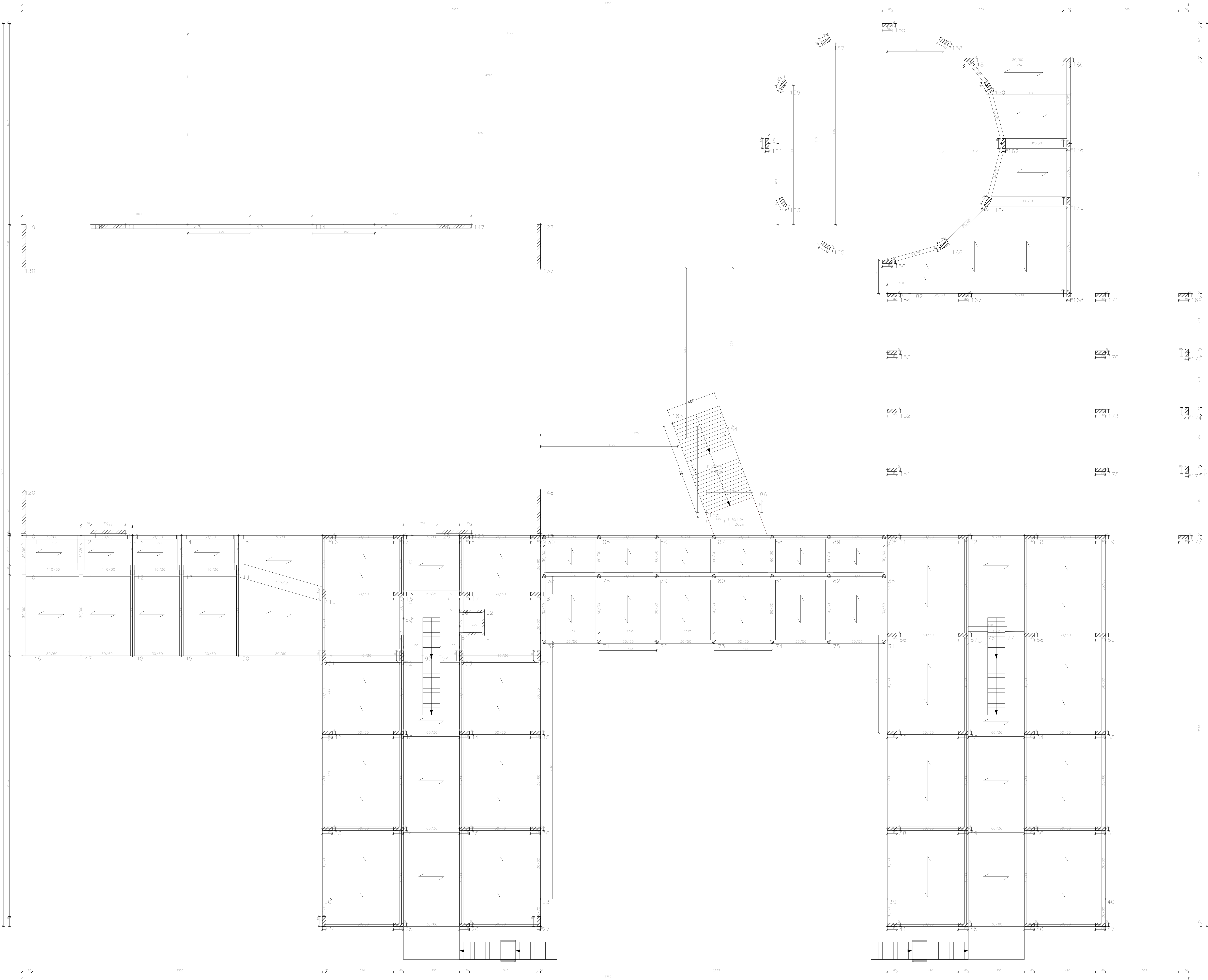
PIANTA IMPALCATO QUOTA m: 4.92
